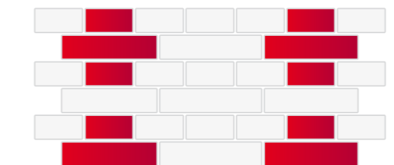
WIĄZANIE KRZYŻOWE TYP 1
