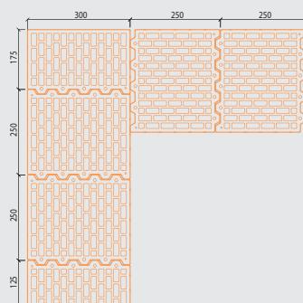
Pierwsza warstwa
