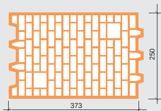
Przekrój pustaka Porotherm 25 Profi
