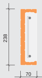
Przekrój belki nadprożowej 23.8
