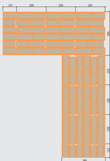
Schemat narożnika
