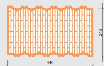
Przekrój pustaka Porotherm 44 EKO+ Profi
