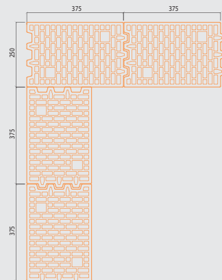
Drua warstwa
