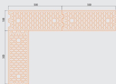
Druga warstwa
