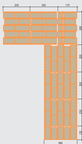
Schemat narożnika
