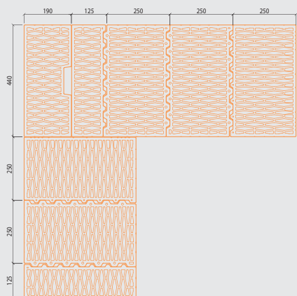
Druga warstwa
