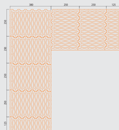
Druga warstwa
