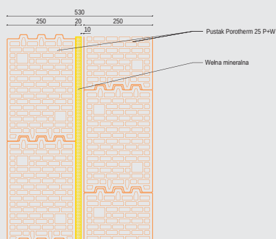
Śchemat ściany podwójnej
