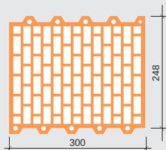
Przekrój pustaka Porotherm 30 P+W
