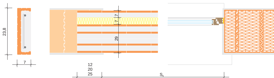
belka nadprożowa 23.8
