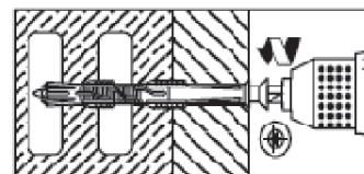
3 Wkręć wkręt w tuleję plastikową
